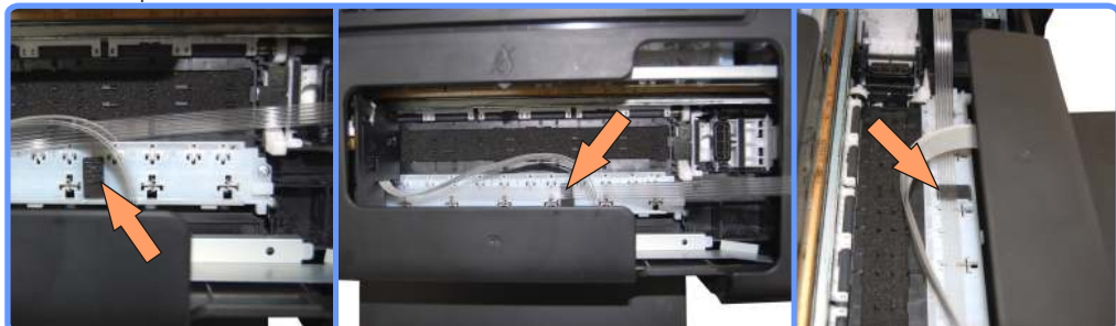
Прокладка шлейфа C110
