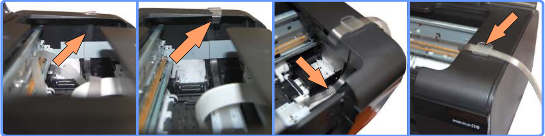
Прокладка шлейфа С110
